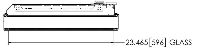
SECTION A-A
