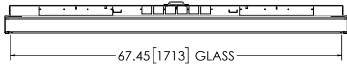
SECTION D-D
